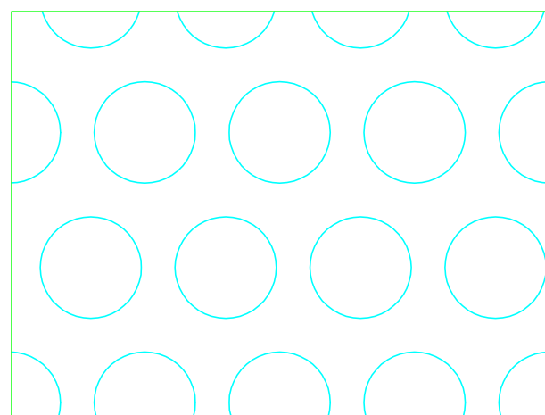
DETALJ A SKALA 1:1 PERFORERAD ALU-PLÅT
